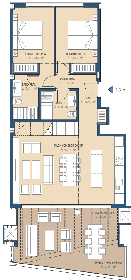
PLANTA TERCERA
